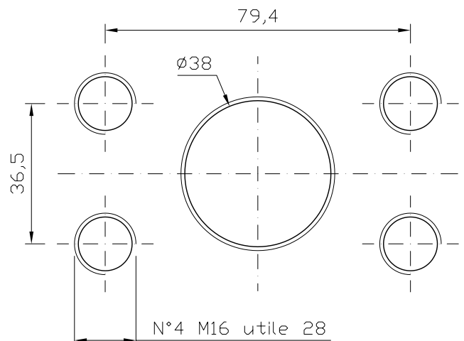
Outlet
