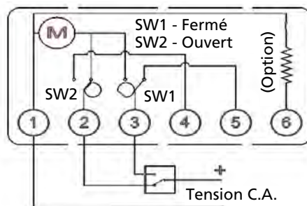
Câblage in-situ
