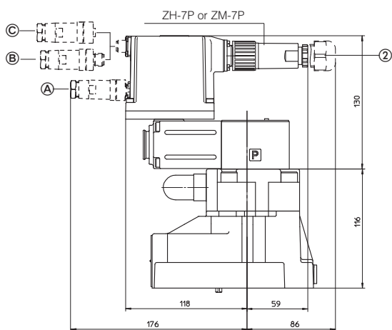
AGMZO-AE-32 (-AES-* dotted line)
