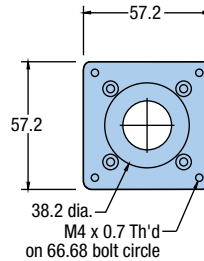
SM 23 or NEMA 23
